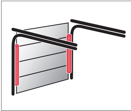
拉簧系统 MyDoor X
